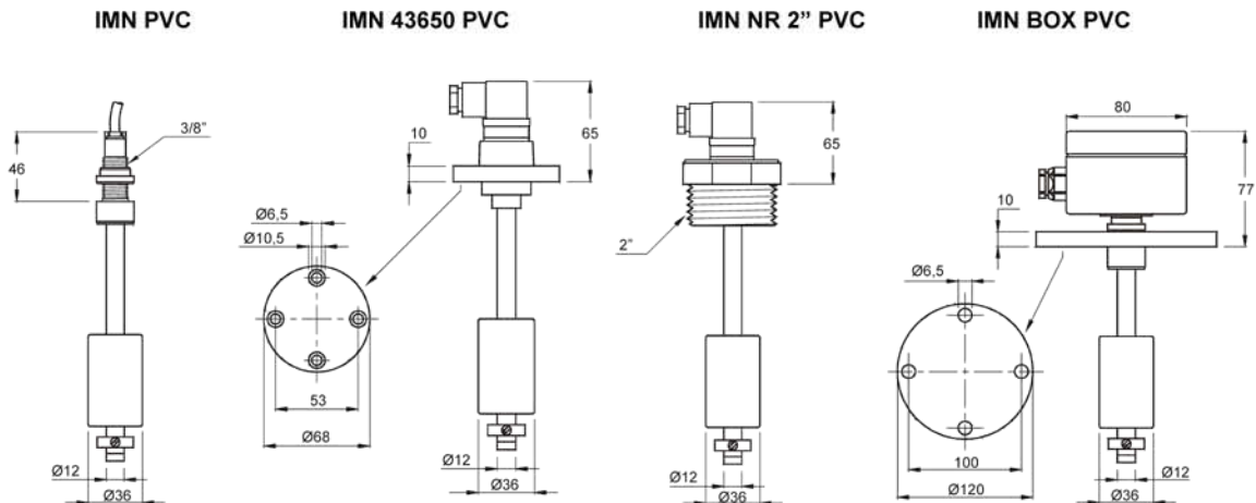
INTERRUPTORES MAGNÉTICOS DE NIVEL. MODELOS Y CARACTERÍSTICAS PARTICULARES. EJECUCIÓN ESPECIAL
